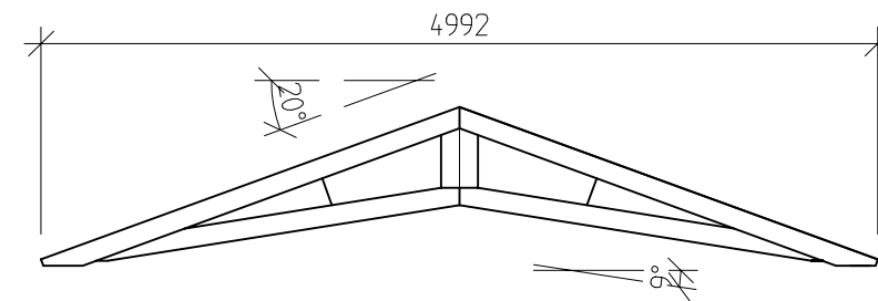
TAKSTOL TYP 2
