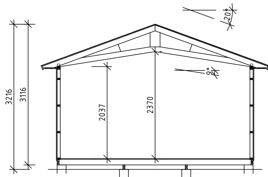
SEKTION
