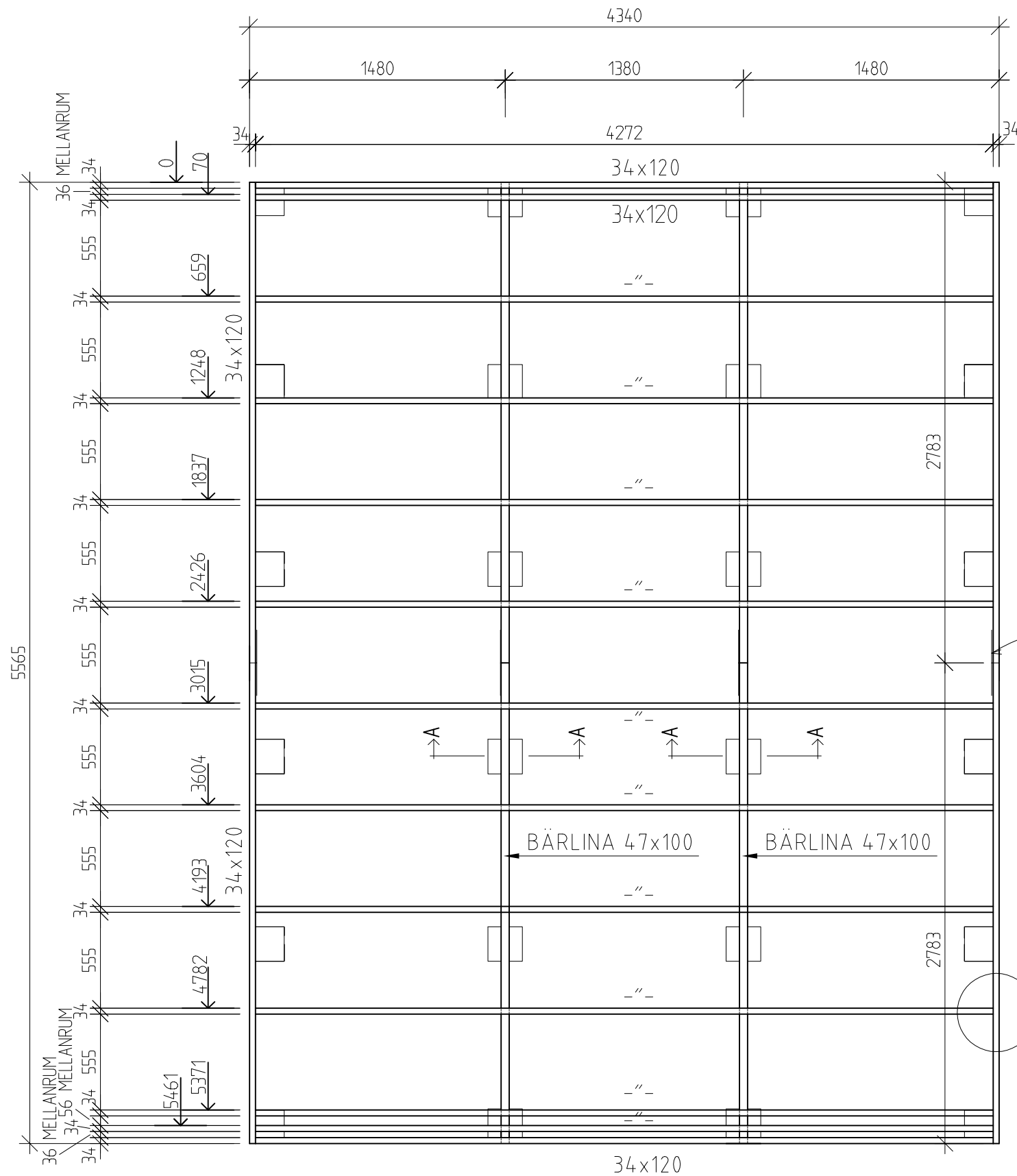
BJÄKLAGSPLAN
