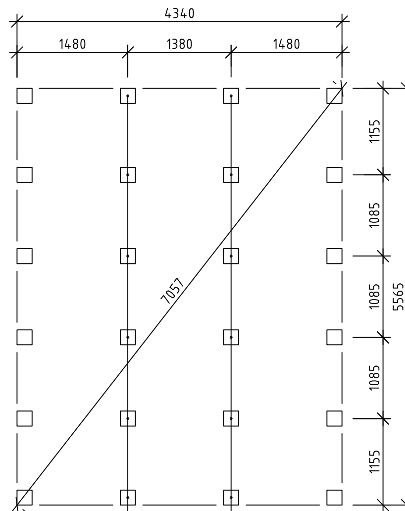
PLINTPLAN
