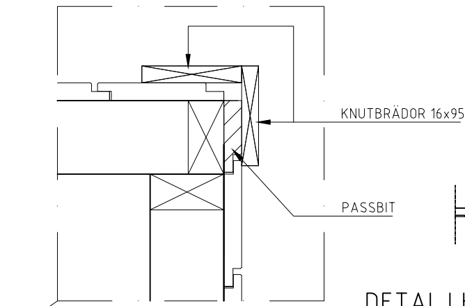
DETALJ HÖRN
