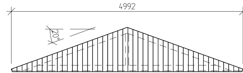
TAKSTOL TYP 1 MED FUNKISPANEL 17x120 mm
