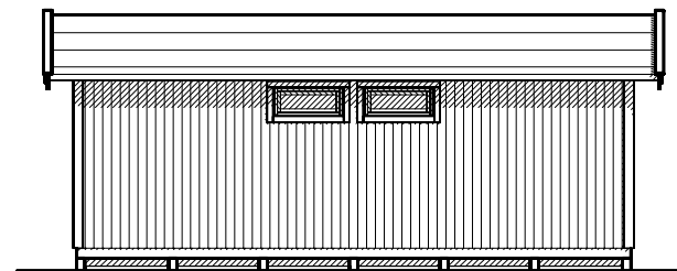
FASAD MOT
