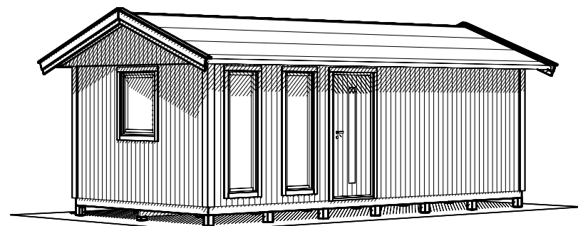
PERSPEKTIV
