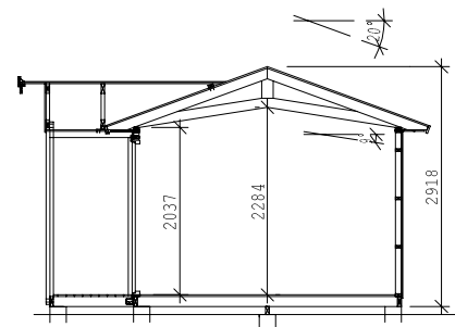
SEKTION
