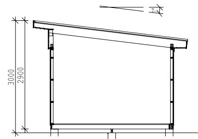
SEKTION
