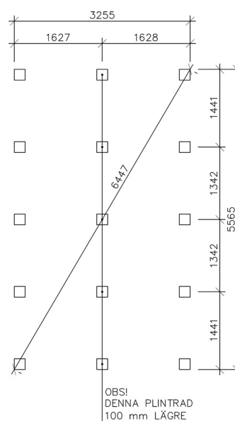
Plintritning
