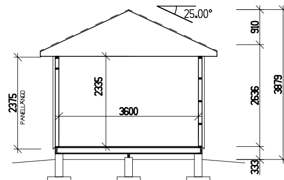
SEKTION
